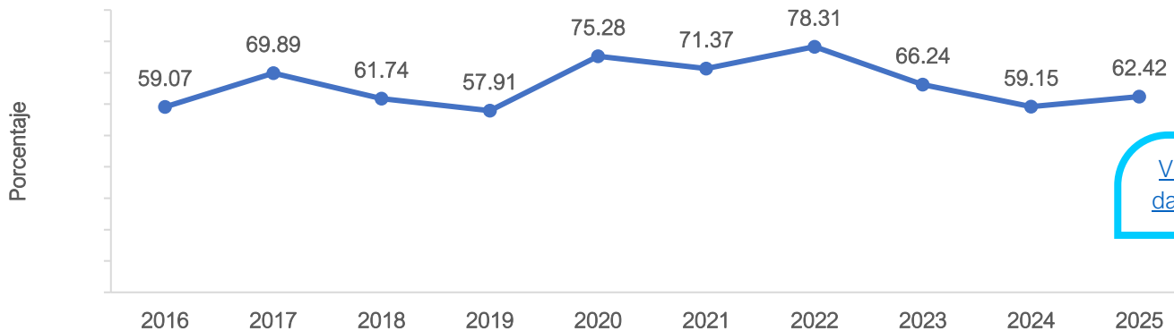
Porcentaje de energía renovable en la generación total de energía eléctrica, 2016 - 2025
